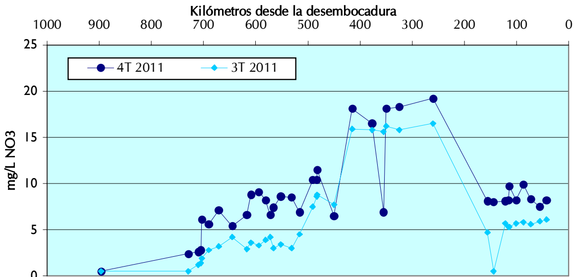
Gráf. 3.4. Evolución de nitratos en el eje del río Ebro
